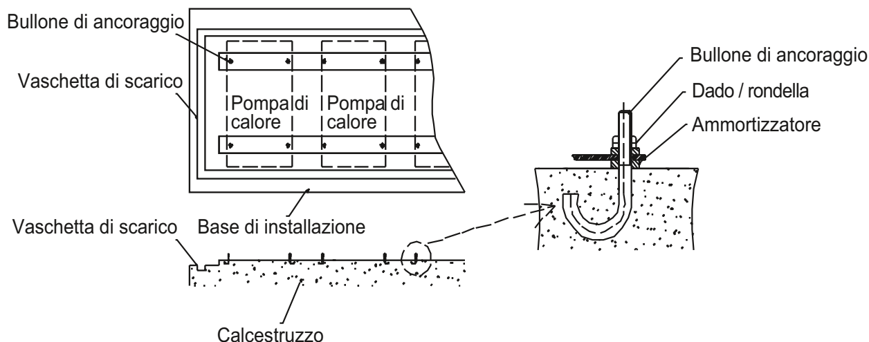
Figura 4. Base di installazione
