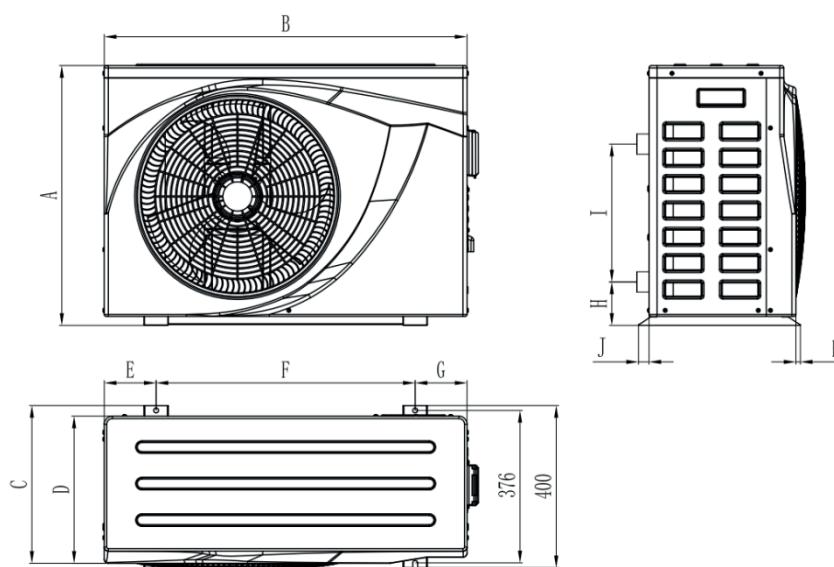
Figura 3. Dimensioni della pompa di calore: TCPO 30 trifase
