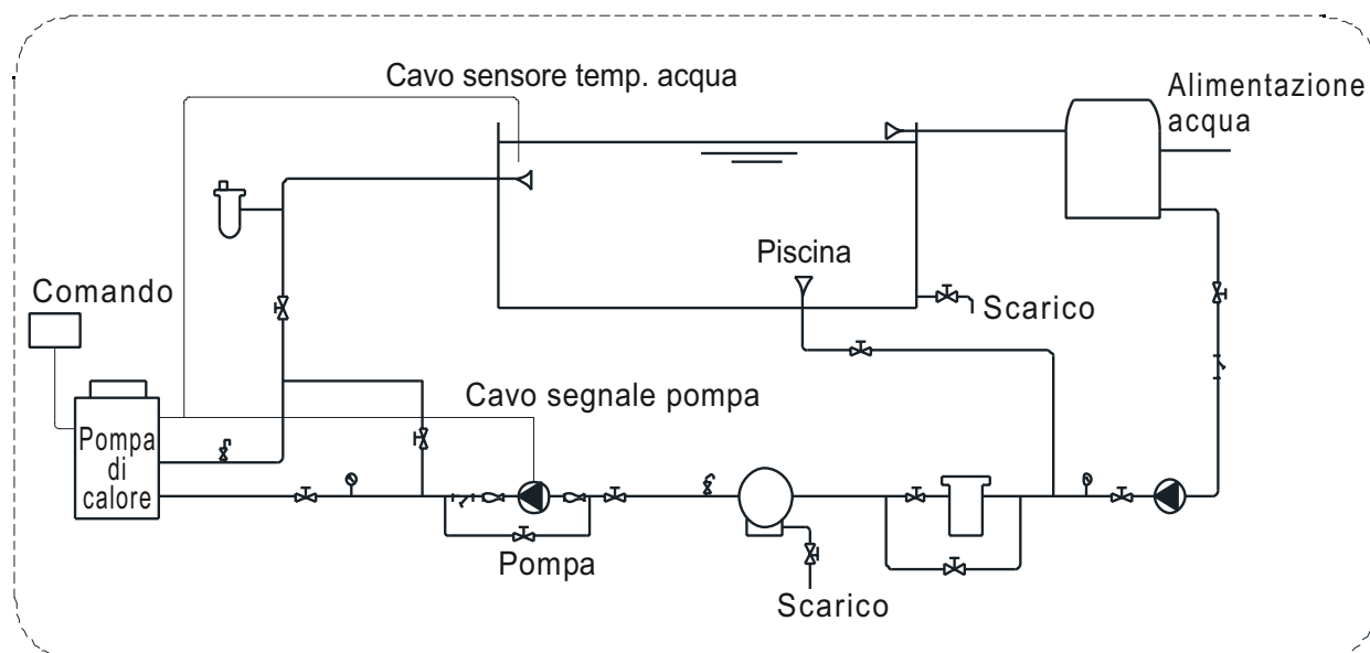
Figura 7 Schema (Singola Unità di riferimento)
