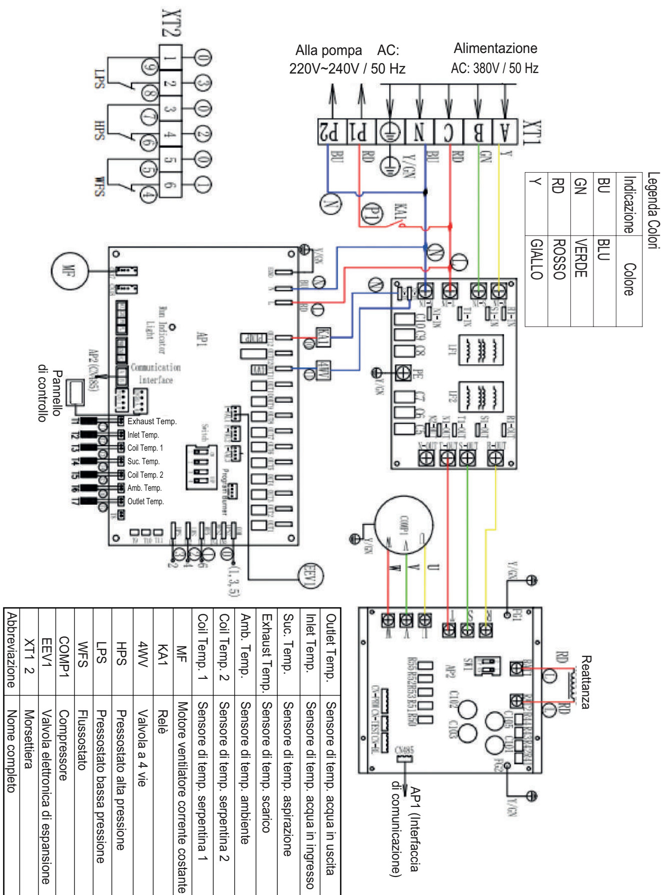
Figura 12 Schema dei cablaggi elettrici
