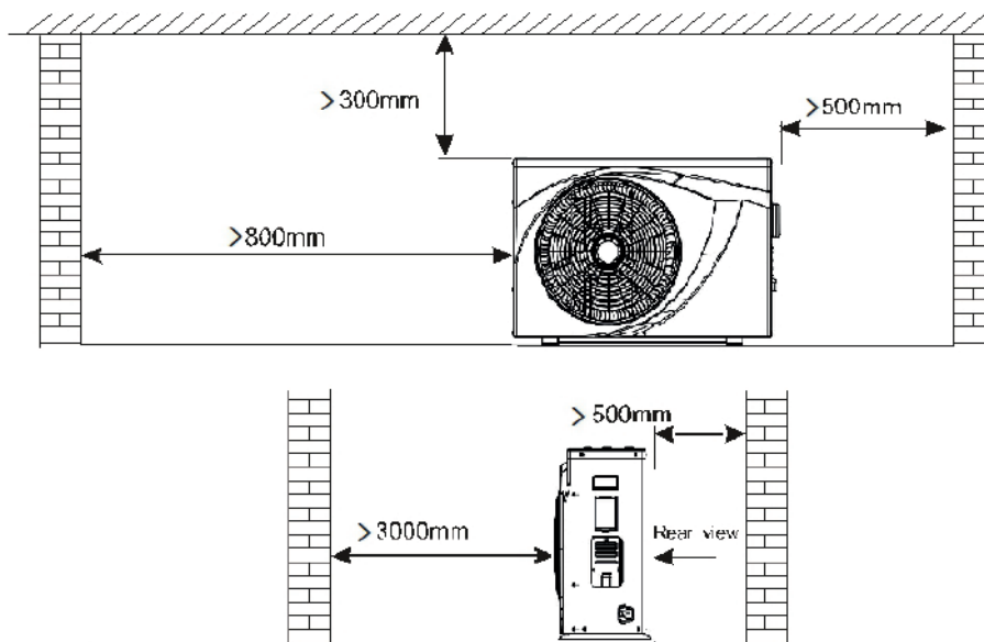
Figura 2. Requisiti di spazi di installazione orizzontale (mm)
